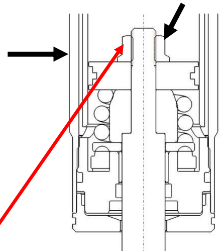
〔 断面図 ナット 〕
