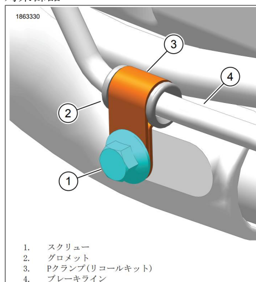
対策部品
