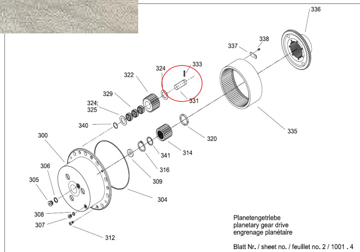
ハブリダクション機構分解図 赤丸: プラネタリギアピン
