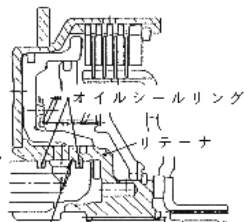
断面拡大図
