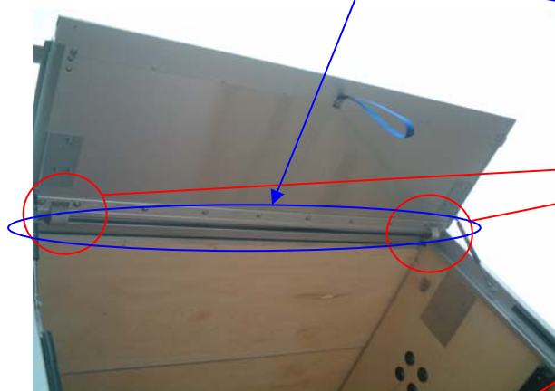
樹脂製ヒンジ (商品名:ラミネートヒンジ)
