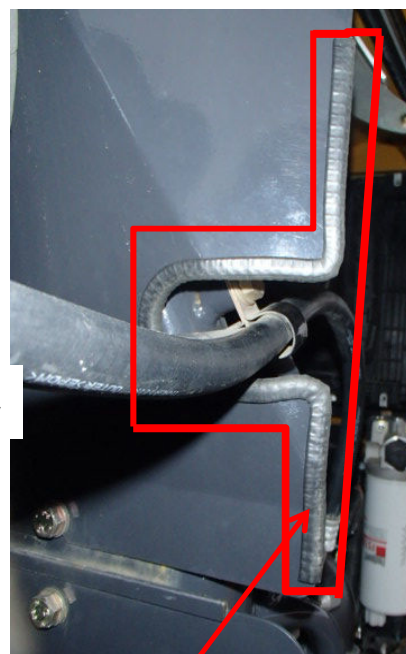
トリムゴムカバーを取付ける
