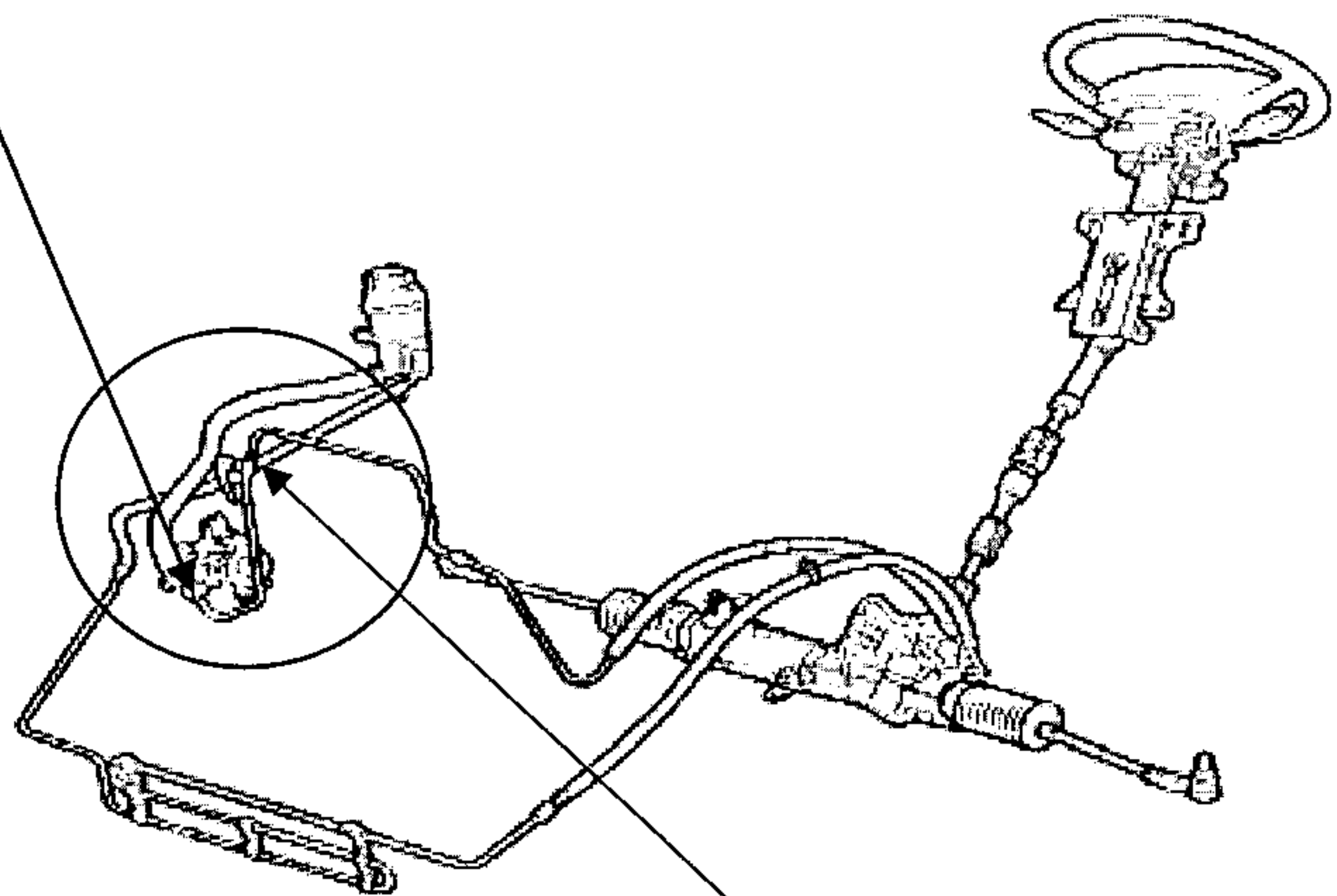
パワーステアリング高圧ホースクランプ
